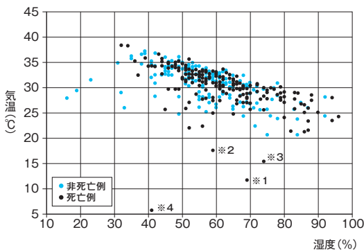
図10 運動時熱中症発生時の相対湿度と気温の関係 (1970~2012年) (中井,2012)
